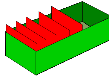
SYSTEM.ADMIN.QMGR.EVENT
